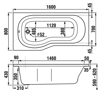
Instalační rozměry vestavné vany
