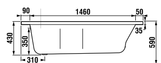
Instalační rozměry vany s panelem
